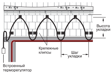
Рисунок 2 Вид на крышу с установленной системой антиобледенения.
