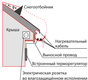
Рисунок 3 Вид сбоку на крышу с установленной системой антиобледенения.
